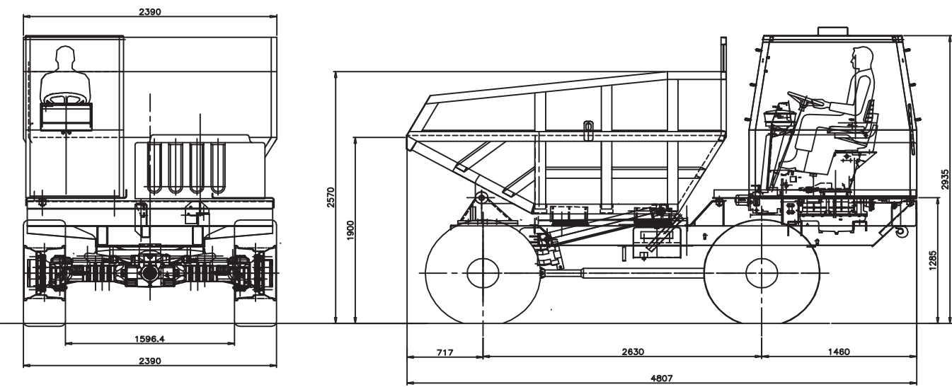
D160 16 ton dumper
