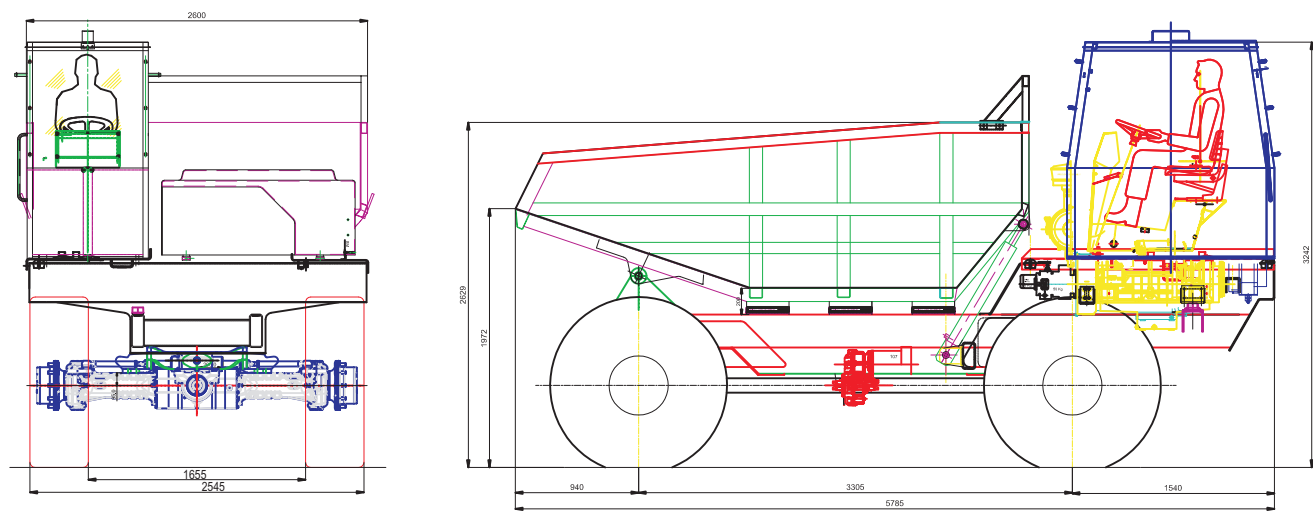
D160 16 ton dumper
